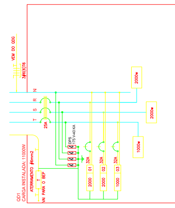
11 DIAGRAMA MULTIFILAR - OD1 SEM ESCALA
